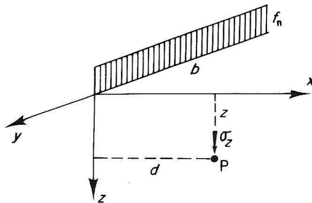
FIG. 5. — Calcul de \sigma_z en un point P du plan Ozx.
