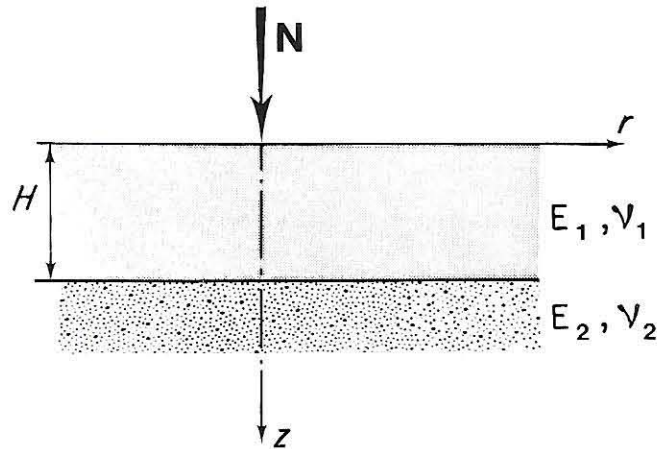
FIG. 1. — Définition du sol et de la charge.
