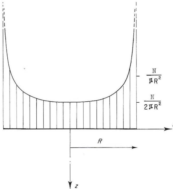
FIG. 1. — Représentation de la charge exercée par une fondation circulaire.
