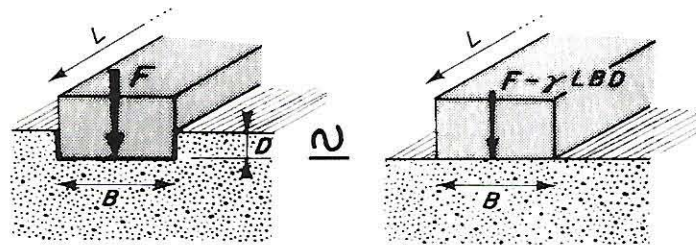
FIG. 6. — Le tassement d'une fondation enfoncée de D (Condition des fondations superficielles : D/B petit) et exerçant une charge de résultante F est généralement considéré comme égal à celui d'une fondation reposant sur le sol arasé à la profondeur D et exerçant la charge F - \gamma LBD ( \gamma : poids volumique moyen du sol enlevé).
