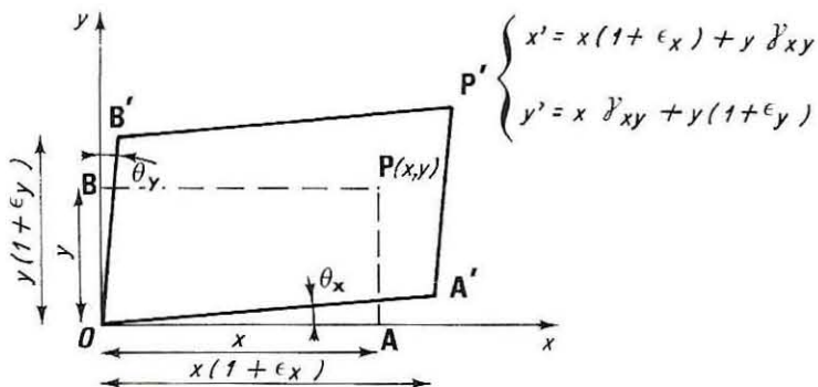
FIG. 2. - Définition des déformations.
