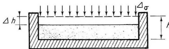
FIG. 2. — Essai de compression oedométrique. Le tiret indique la position initiale de la surface de l'échantillon et le trait plein sa position finale.
