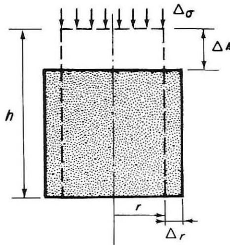
FIG. 1. — Essai de compression simple permettant de mesurer le module d'Young et le coefficient de Poisson. Le tiret indique la forme initiale de l'échantillon et le trait plein sa position finale.
