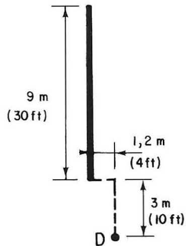
FIG. 7. — Définition de la semelle filante de l'exemple 2.
