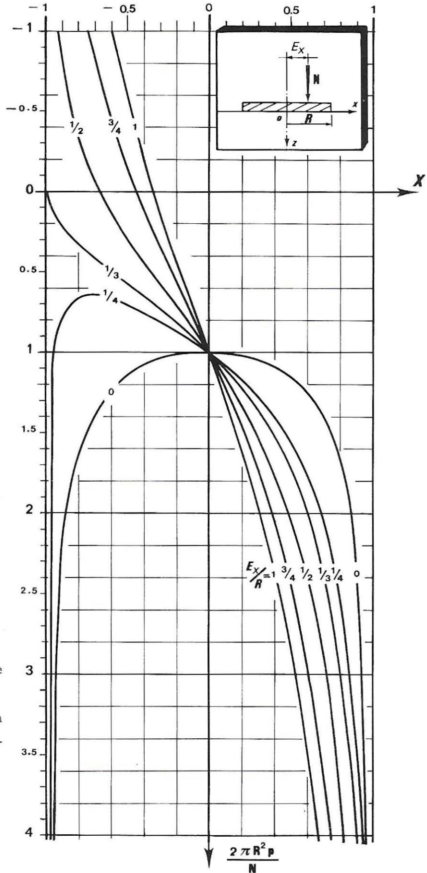
FIG. 1. — Coupe par le plan Ozx de la distribution de la charge p pour diverses valeurs de l'excentricité. On voit que lorsque la charge est appliquée à l'extérieur du tiers central la fondation se décolle du sol. La distribution indiquée n'est alors plus valable. Si la charge était uniformément répartie la limite serait constituée par le quart central.
