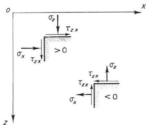
FIG. 1. - Conventions de signe des contraintes.
