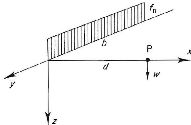
FIG. 2. — Calcul du tassement d'un point P de l'axe Ox.
