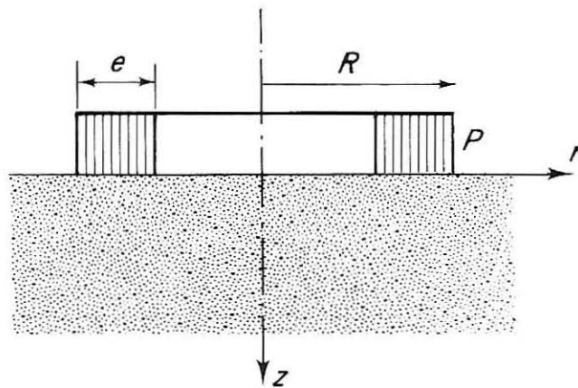
FIG. 1. — Définition de la charge annulaire uniforme.
