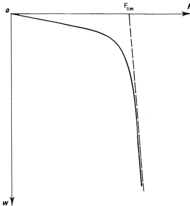
FIG. 3. — Courbe de l'enfoncement en fonction de la charge (Il ne s'agit bien entendu que d'un tracé schématisé donnant l'allure moyenne des courbes expérimentales).
