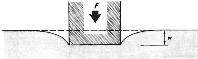
FIG. 2. — Tassement w dû à l'application d'une charge F sur le sol. La surface du sol avant application de la charge est représentée par un tiret.
